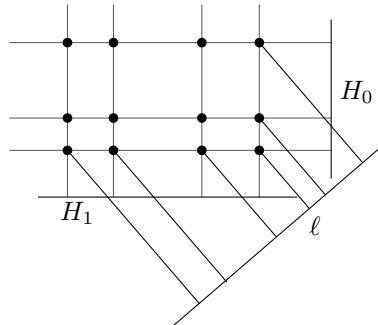
Fig. 6. The proof of Lemma 6.
